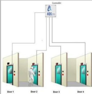
Door Interlocking System
