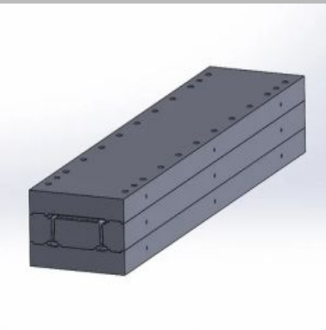
FRP Cable Tray Pultrusion Die
