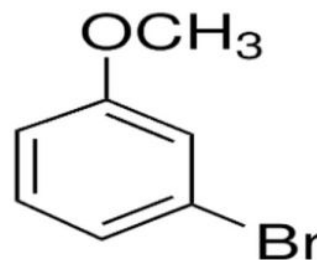
Meta Bromoanisole
