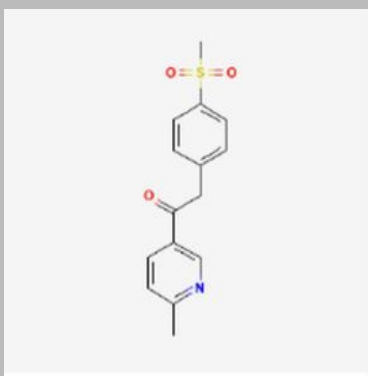
Ketosulphone
