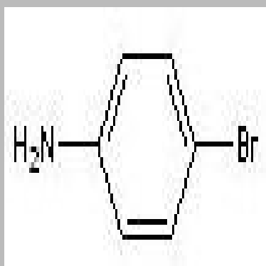
4-Bromoaniline
