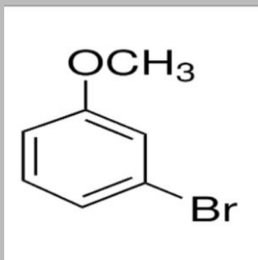
Meta Bromoanisole
